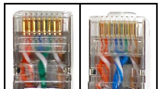
Twisted Pairs
